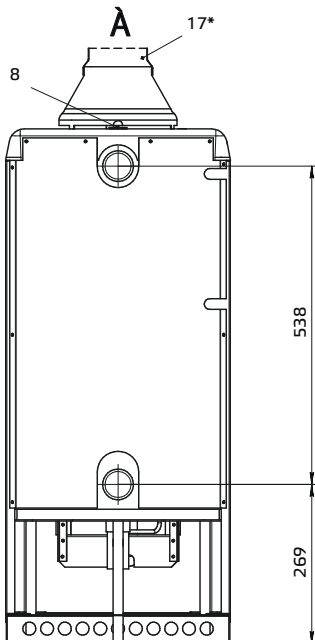
Рисунок 1 — Аппарат отопительный газовый бытовой одноконтурный
